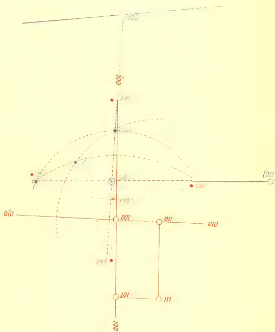
11. Анортитъ.
